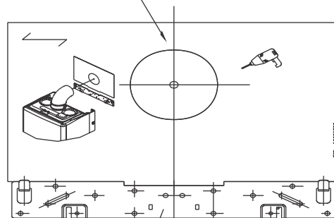
Plantilla de Marcado (Sólo modelos Tiro Balanceado)
